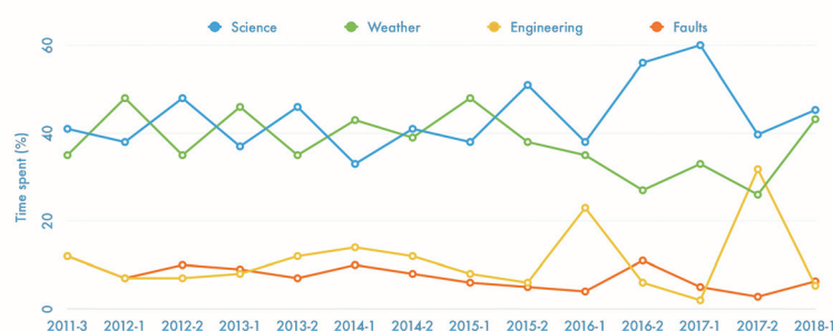
SALT time usage per semester
